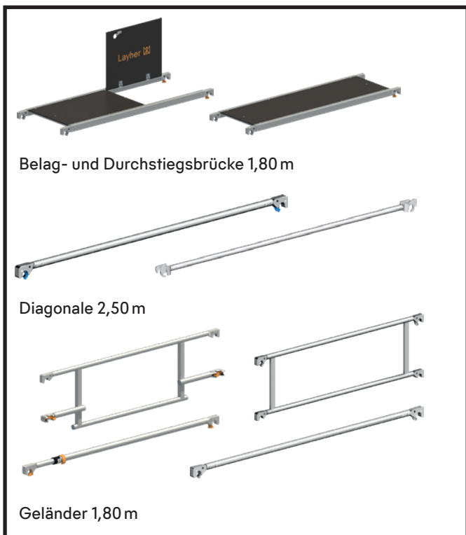
Arbeitsfläche 0,75 x 1,80 m - Zifa, Uni Leicht
